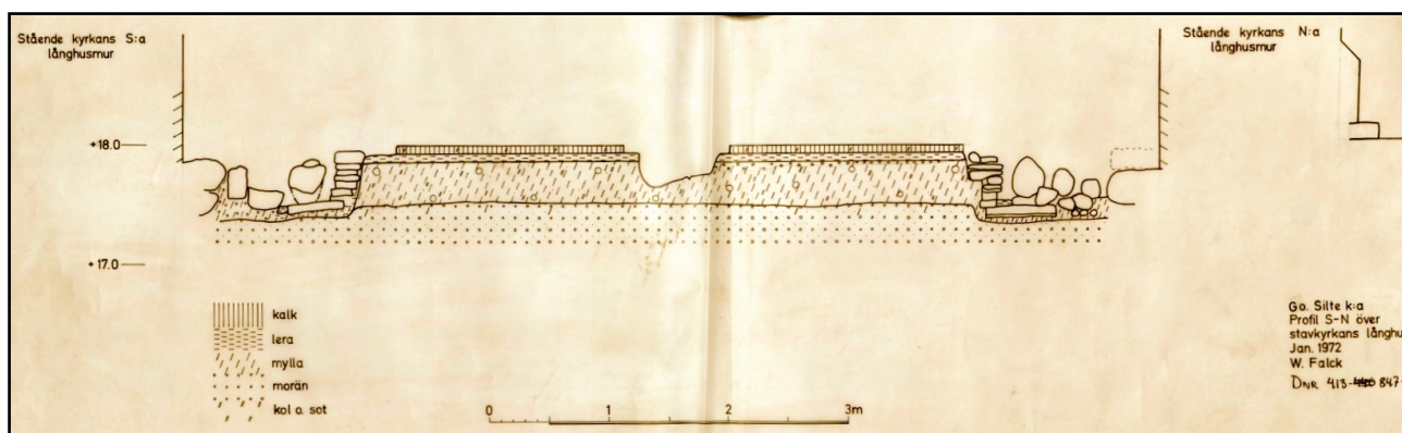
(Fig.6) Tvärprofil av stavkyrkans grund mot väster. Ritad av W Falck, 1972 (ATA).
