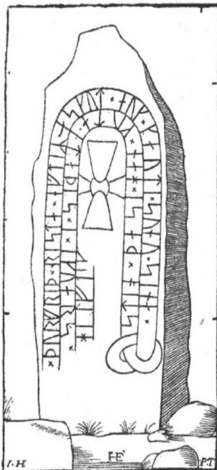
B. 857.
